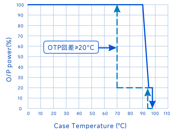
输出功率Vs.壳温（BH机型）
